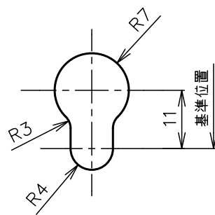
アース穴詳細図 (S=1:1)
