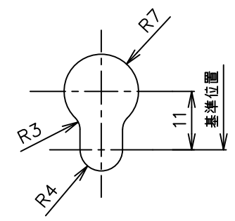
アース穴詳細図 (S=1:1)
