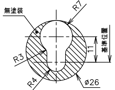
アース穴詳細図 (S=1:1)
