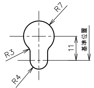
アース穴詳細図 (S=1:1)
